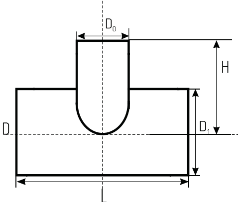
ТРОЙНИК ( D/D_0/D_1 ; L=l , H=h )
